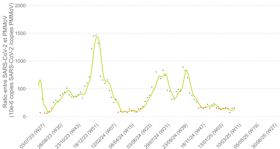
Ratio entre SARS-CoV-2 et PMMoV agrégées au niveau national.
