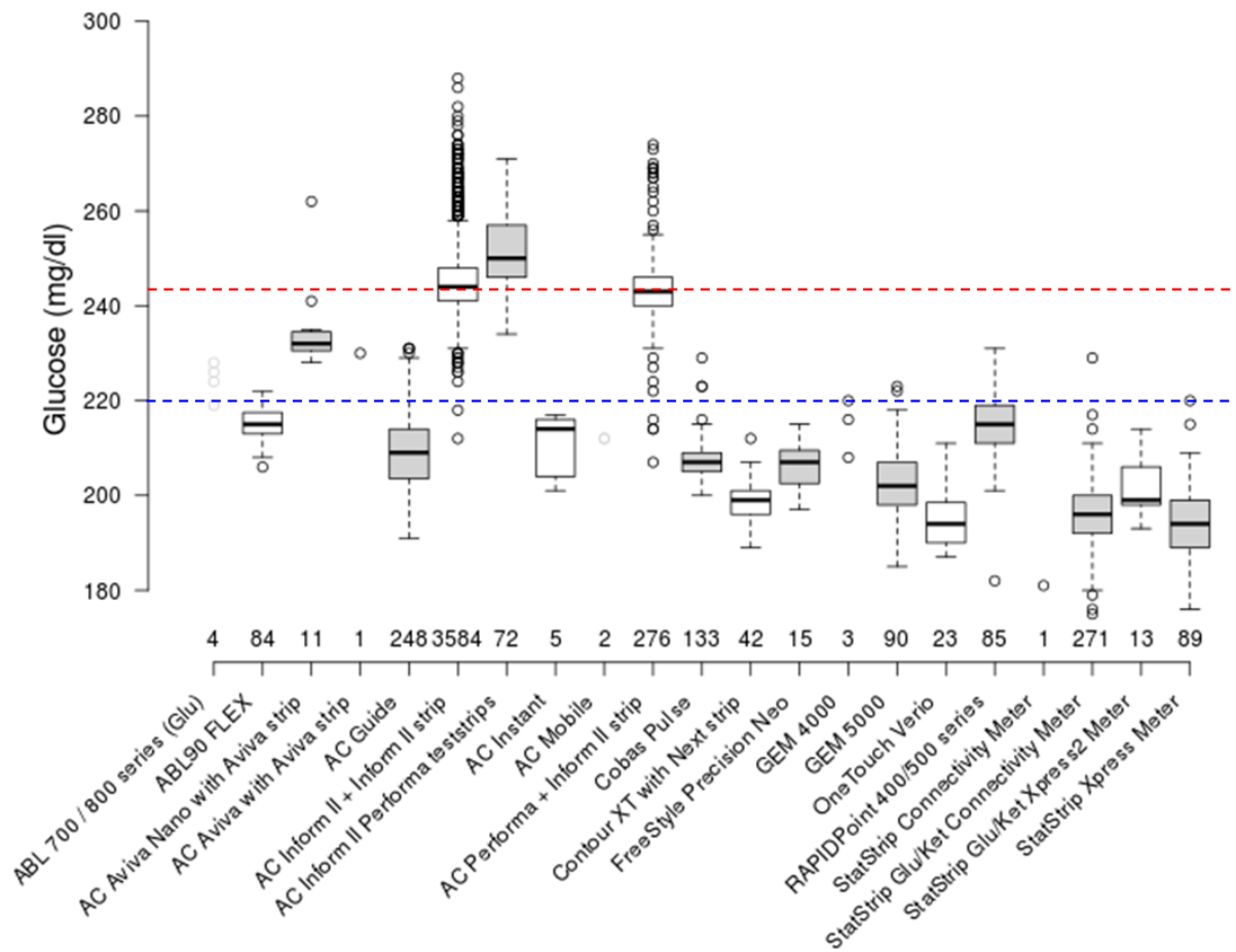
Figure 1. Distribution de l'ensemble des résultats par glucomètre. Le trait pointillé bleu représente la valeur de référence mesurée par la méthode à l'hexokinase (219.79mg/dL); le trait pointillé rouge représente la valeur médiane globale (243mg/dL). AC = Accu-Check.
