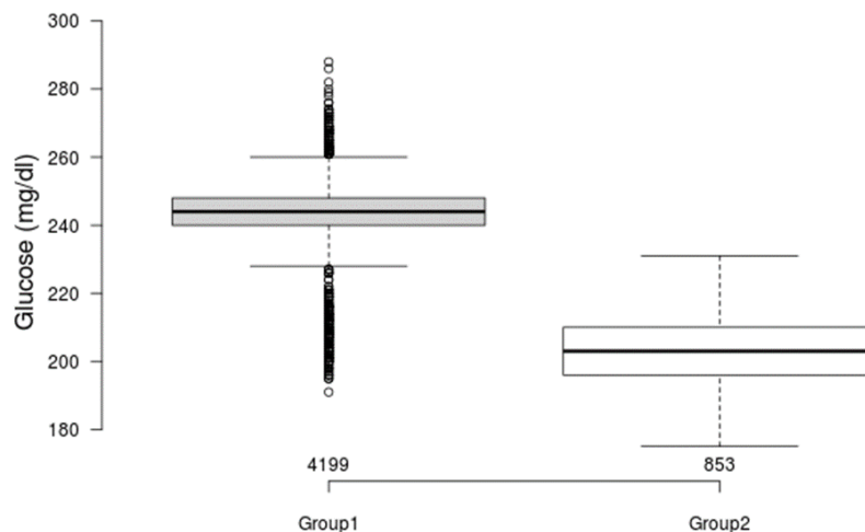
Figure 3. Comparaison des résultats au sein des deux populations observées. Groupe1 : médiane=244mg/dL, SD^*=5.93 , CV^*(\%)=2.43 . Groupe2 : médiane=203mg/dL, SD^*=10.38 , CV^*(\%)=5.11 . Les deux groupes présentent des médianes statistiquement différentes (Wilcoxon/Mann-Whitney, P<0.01 ). Groupe1 : Accu-Check serie – Groupe2 : ABL700/800, ABL 90Flex, Cobas Pulse, Contour XT, FreeStyle serie, GEM 4000, GEM 5000, One Touche Verio, Rapid Point, StatStrip serie.
