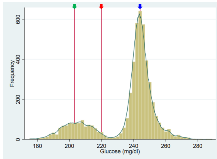
Figure 2. Distribution de l'ensemble des résultats belges (n=5048). La ligne horizontale supérieure désigne le nombre de participants dans la barre la plus élevée. La flèche rouge indique la valeur de référence mesurée par la méthode à l'hexokinase (219.79mg/dL); la flèche bleue indique la valeur médiane de la population 1 (244mg/dL), la flèche verte indique la valeur médiane de la population 2 (203mg/dL). L'estimation de la densité de probabilité a été réalisée par la méthode du noyau (kernel density plot).
