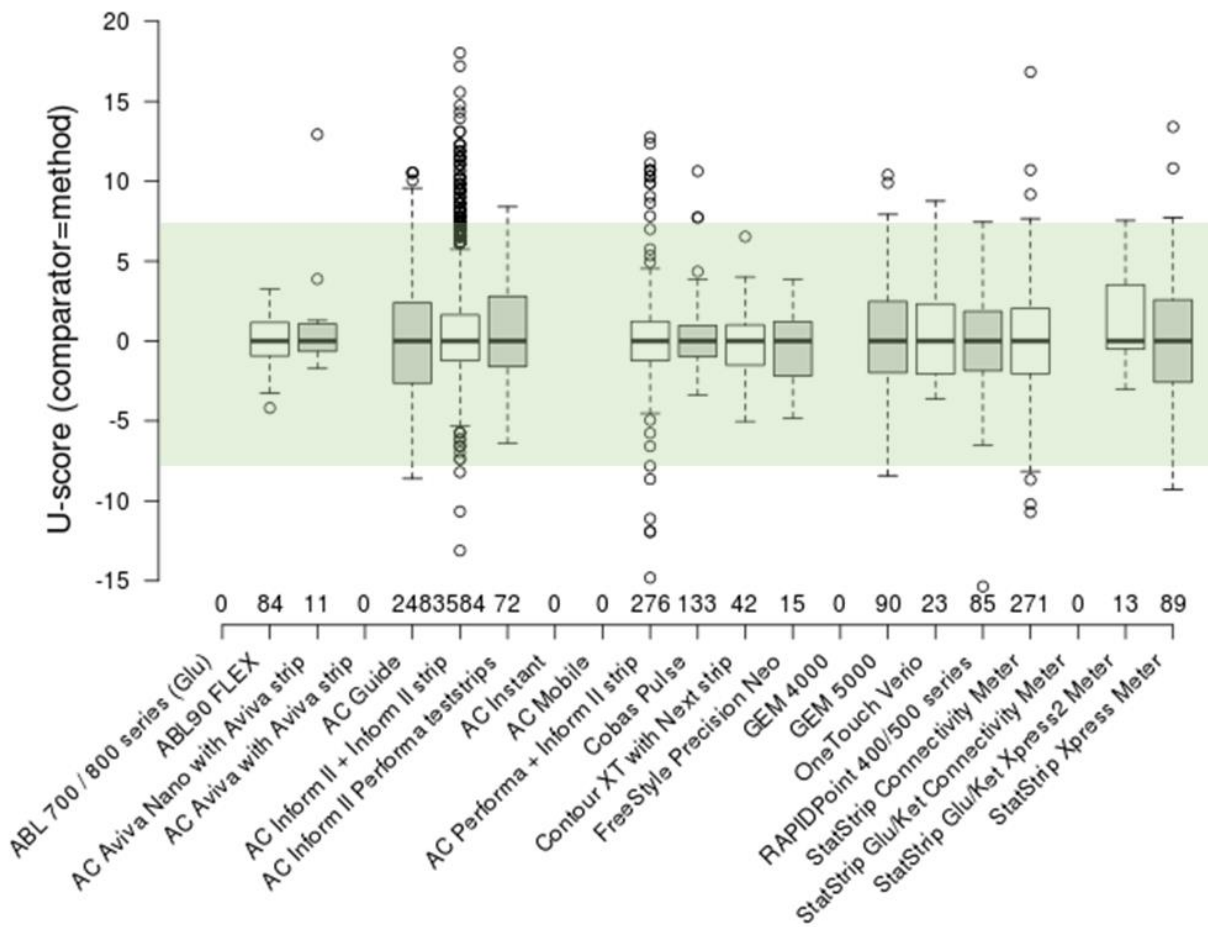
Figure 6. Distribution de l'ensemble des U-scores (%) par type de glucomètre ( U_m ). La zone verte, |U_m| \leq d (6.9%). AC = Accu-Check.
