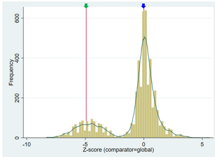
Figure 5. Distribution de l'ensemble des Z_g belges ( n=5048 ). La ligne horizontale supérieure désigne le nombre de participants dans la barre la plus élevée. La flèche bleue indique la valeur médiane de la population 1 ( -0.00 ), la flèche verte indique la valeur médiane de la population 2 ( -4.92 ). L'estimation de la densité de probabilité a été réalisée par la méthode du noyau (kernel density plot).
